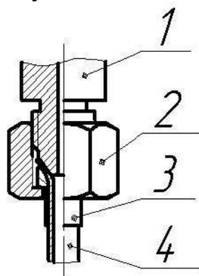
Рисунок 1 – Подсоединение прибора к трубопроводу 1 – штуцер прибора; 2 – гайка; 3 – ниппель; 4 – медная трубка.
